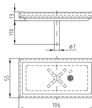
Skilte-grundplade med stift til påsvejsning.
