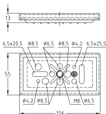
Grundplade med gevindtilslutning.
