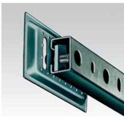
Justering af knopperne på bagsiden sørger for at holde grundpladen i rigtig position ved rækkemontage på en MPC-systemskinne.
